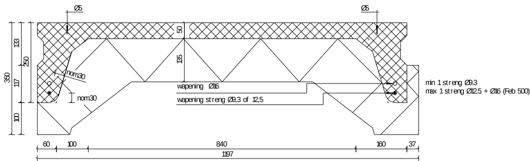
Type R350/ 12/ 3.0
