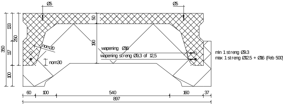
Type R350/ 0.9/ 3.5
