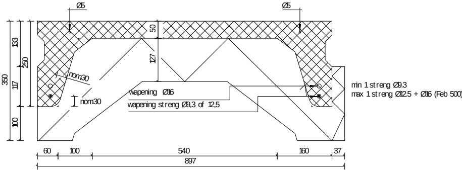
Type R350/ 0.9/ 3.0
