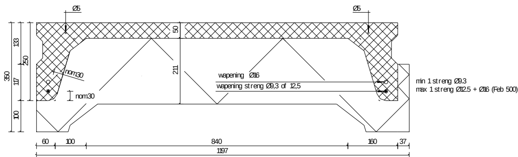
Type R350/ 12/ 4.0
