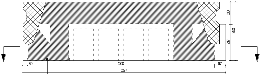
Aanzicht kop
