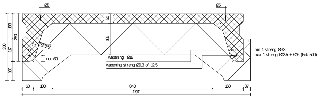
Type R350/ 12/ 3.5
