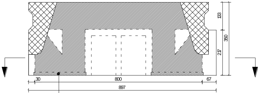
Aanzicht kop
