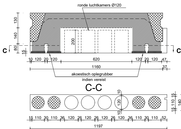
Aanzicht kopzijde L1200
