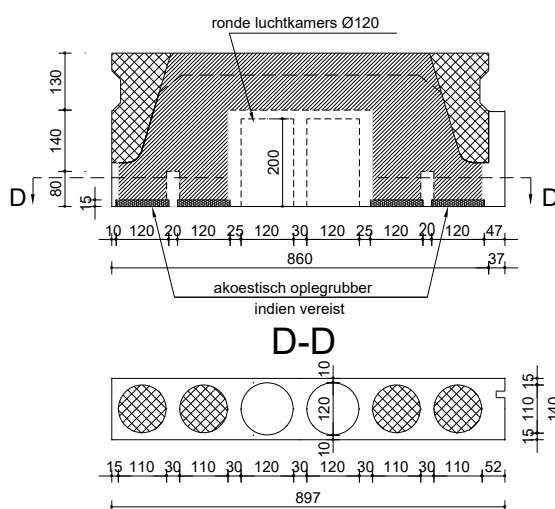
Aanzicht kopzijde L900
